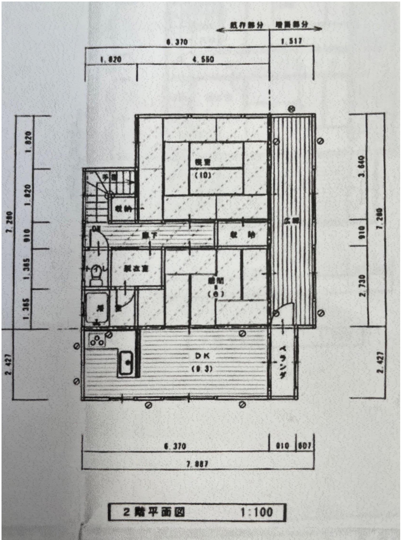
間取り図 (2階住居)
